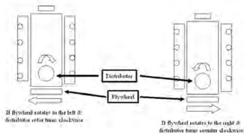
CCW Rotation
